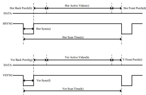
图 4-2 摄像头数据包输出时序
