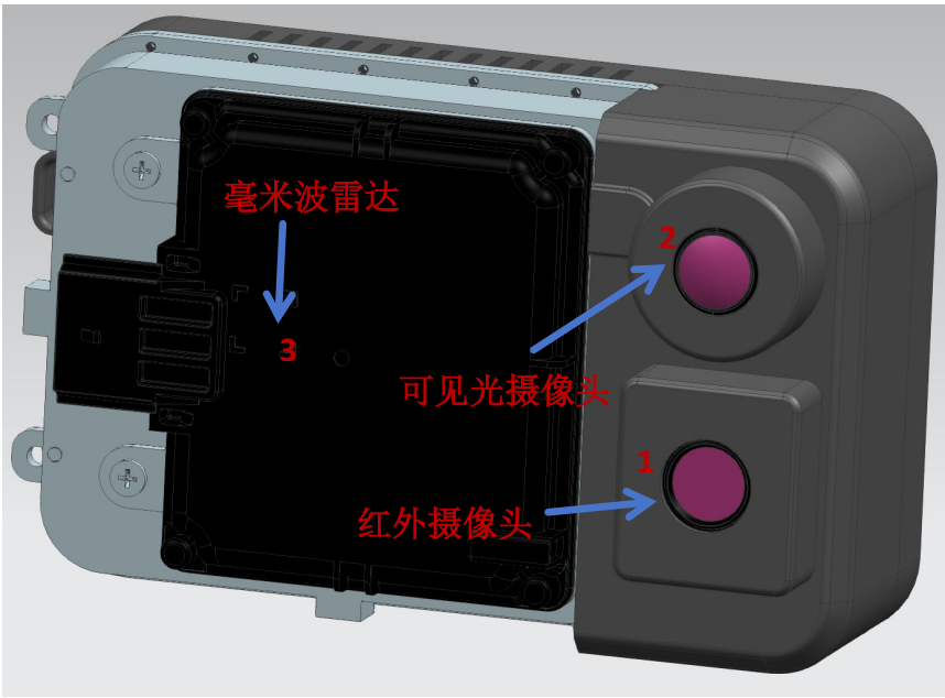
图 2-1 产品正等测图
